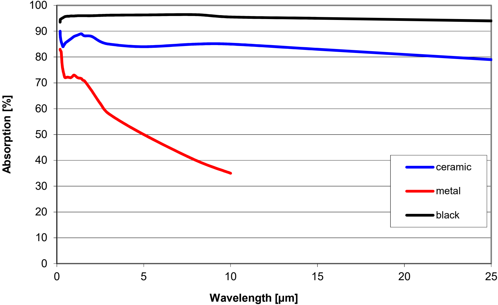
Absorption 190nm - 25μm
